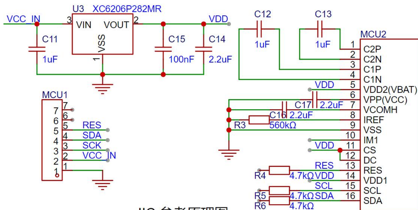
IIC 参考原理图
