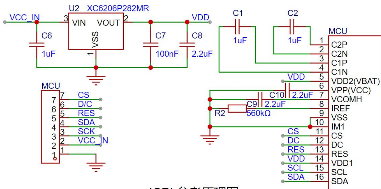
4SPI 参考原理图
